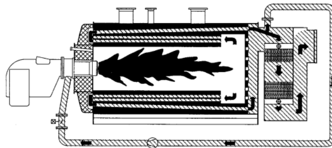
图3 外部烟气循环系统
